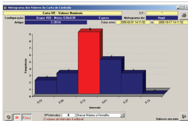
Figura 3 - Histograma de frequência no EGITRON SPC Pro
