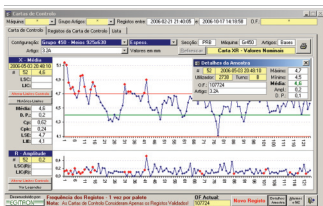
Figura 1 - Visualização de uma carta de controlo XR a partir do EGITRON SPC Pro
